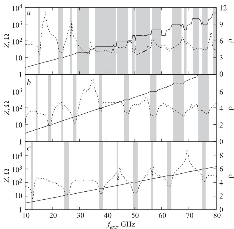
Рис. 1. Амплитуда импеданса (пунктирная линия) и число вращения (сплошная линия) при изменении частоты внешнего сигнала для различных частот внешнего резонатора: 17.3 GHz ( a ), 34.6 GHz ( b ), 69.2 GHz ( c ). Добротность внешнего резонатора Q = 750 , напряжение питания V_0 = 510 mV, амплитуда внешнего сигнала V_m = 20 mW.
