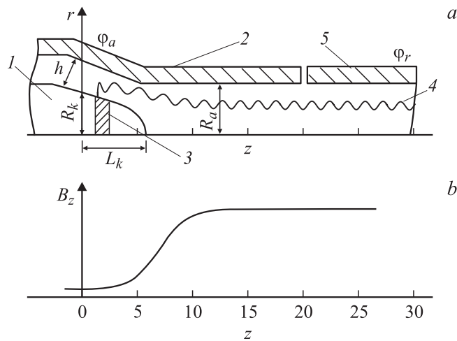
Рис. 1. a — схема магнетронно-инжекторной пушки: 1 — катод, 2 — ускоряющий электрод с потенциалом \phi_a , 3 — эмитирующий пояс, 4 — электронный поток, 5 — тормозящий электрод с потенциалом \phi_r , L_k = 17.8 mm, R_k = 7.4 mm, h = 3 mm, R_a = 8.4 mm. Размеры, указанные на рисунке, нормированы на величину h , масштаб по горизонтальной и вертикальной осям не совпадает. b — распределение продольной составляющей магнитного поля B_z в пространстве дрейфа; c , d , e , f — фазовые портреты пучка в координатах (z, v_z) для различных моментов времени ( t_1 < t_2 < t_3 < t_4 ). Стрелками ( c ) отмечены область торможения частиц из-за магнитной ловушки (стрелка I ) и область ВК (стрелка VC ).
