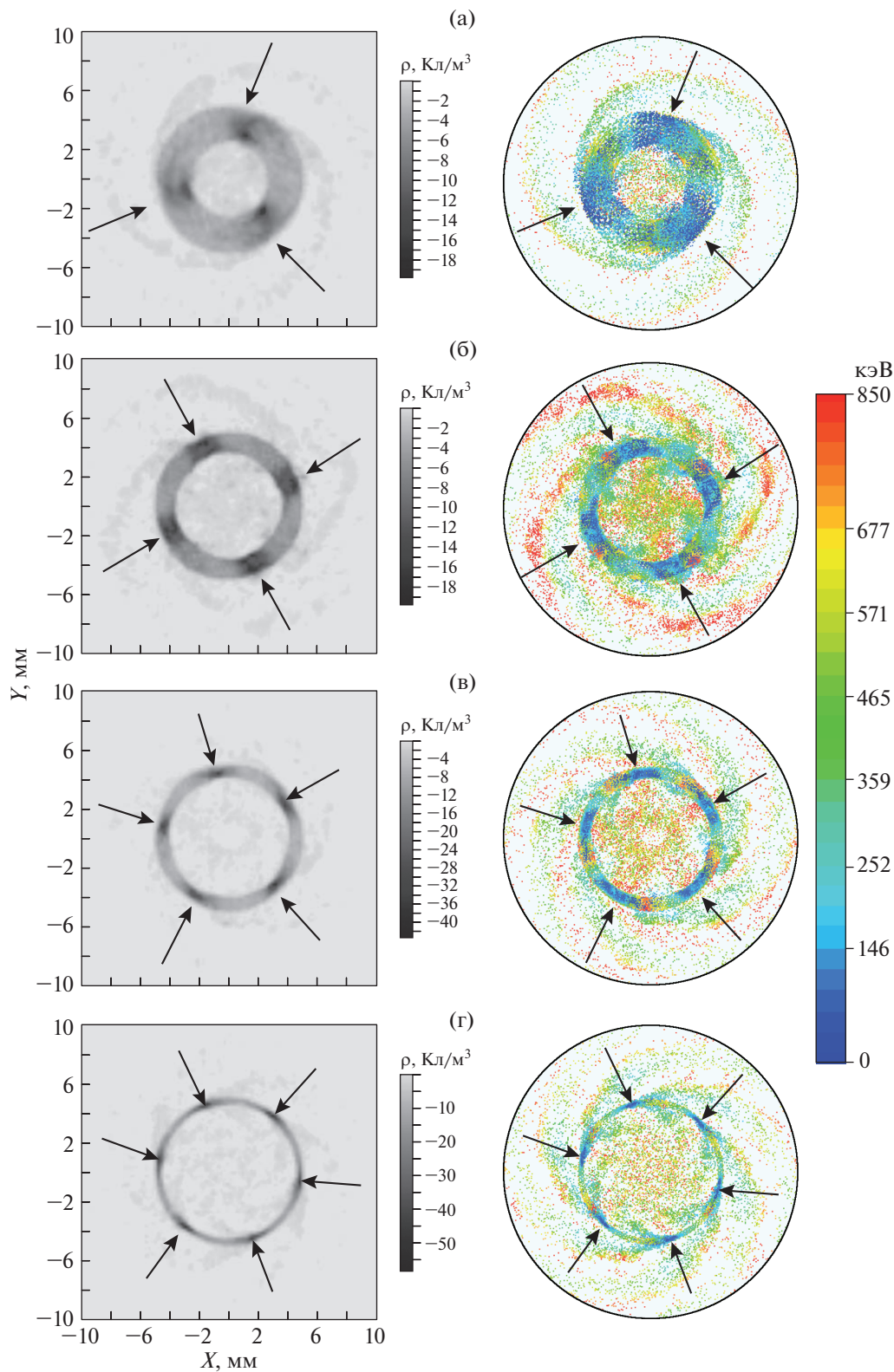
Рис. 3. Распределения плотности пространственного заряда в сечении плоскостью XY в области ВК для режимов с различным количеством N электронных сгустков и соответствующие им конфигурационные портреты пучка. Стрелками показаны электронные сгустки. Режим с N = 3 (при B_0 = 0 Тл и d = 2.5 мм) (а), N = 4 ( B_0 = 0 Тл, d = 1.5 мм) (б), N = 5 ( B_0 = 0 Тл, d = 1 мм) (в), N = 6 ( B_0 = 0 Тл, d = 0.5 мм) (г).
