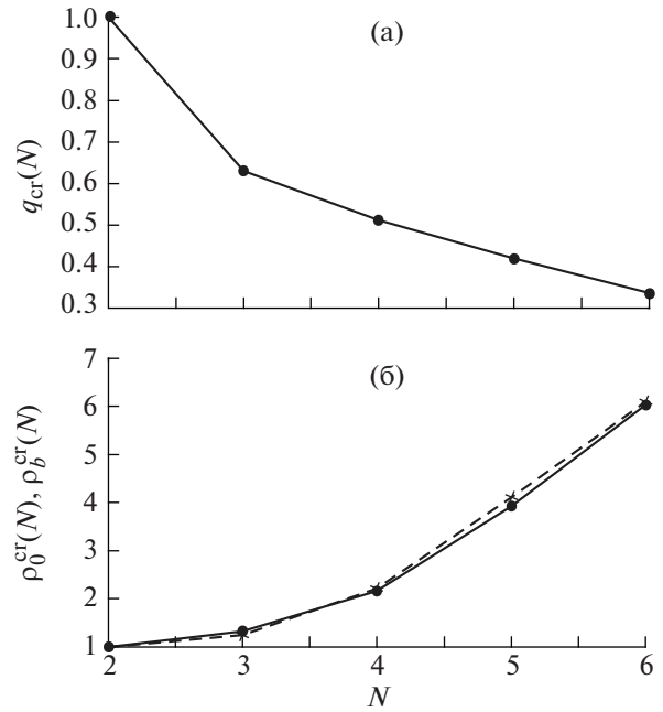
Рис. 5. Зависимость критического заряда в сгустке q_{cr}(N) от номера режима N , нормированная на q_{cr}(N=2) (а). Зависимости (б): непрерывная линия — зависимость невозмущенной критической плотности ПЗ \rho_0^{cr}(N) от количества электронных сгустков N , нормированная на \rho_0^{cr}(N=2) ; штриховая линия — зависимость критической плотности ПЗ в сгустке \rho_b^{cr}(N) от количества электронных сгустков N , нормированная на \rho_b^{cr}(N=2) . Величина индукции внешнего магнитного поля фиксирована и равна B_0 = 1.85 Тл для обоих фрагментов.
