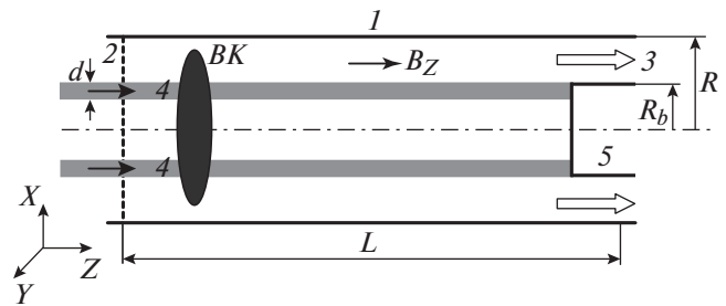
Рис. 1. Схема исследуемой модели: I – цилиндрическая камера дрейфа, 2 – плоскость инжекции электронного потока, 3 – коаксиальный волноводный порт, 4 – кольцевой моноскоростной релятивистский электронный поток, 5 – цилиндрический коллектор.
