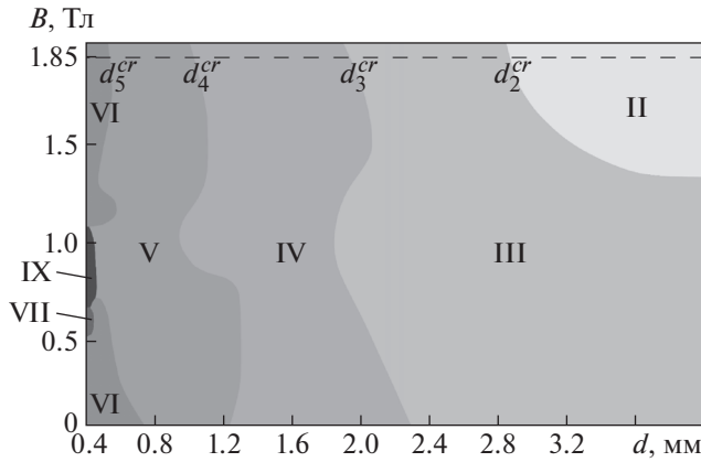
Рис. 4. Карта характерных режимов динамики РЭП на плоскости управляющих параметров “толщина пучка d — индукция внешнего магнитного поля B_0 ”. Градиентом серого выделены области с различным количеством N электронных сгустков. Римскими цифрами обозначено количество электронных сгустков в азимутальном направлении. Зависимость на рис. 5 построена при параметрах, соответствующих штриховой линии; d_2^{cr} , d_3^{cr} , d_4^{cr} , d_5^{cr} — критические величины толщины пучка для режимов N = 2-5 .
